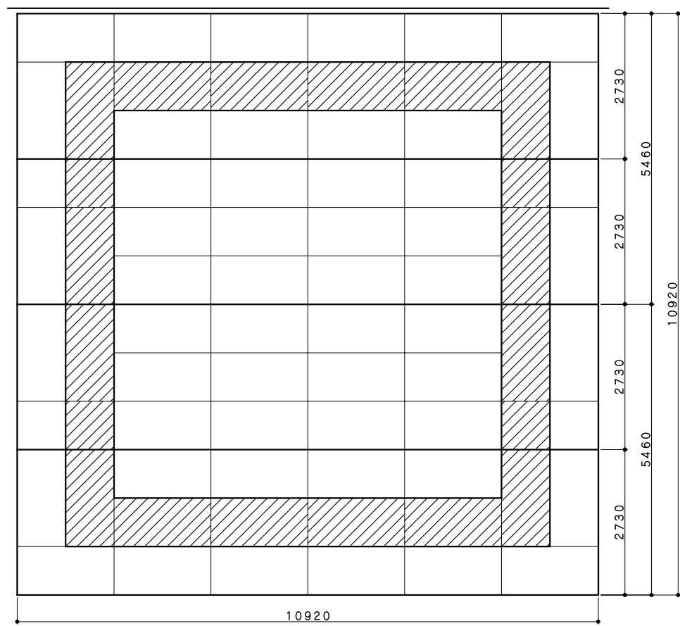
平面図 (72帖 略式サイズ)
