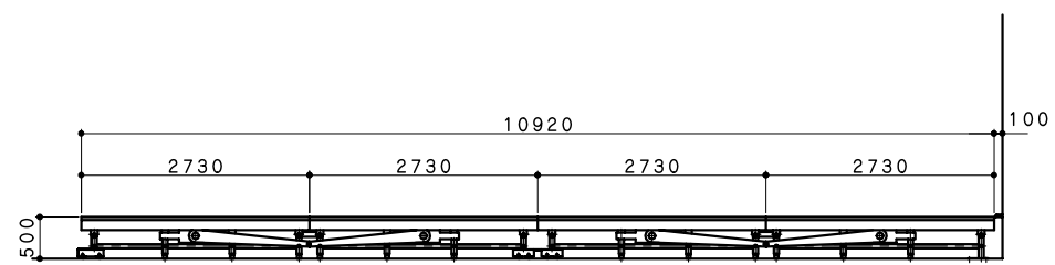
展開側面図 (72帖 略式サイズ)
