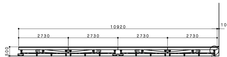
展開側面図 (72帖 略式サイズ)
