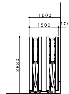
収納側面図 (72帖 略式サイズ)
