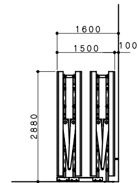
収納側面図 (72帖 略式サイズ)
