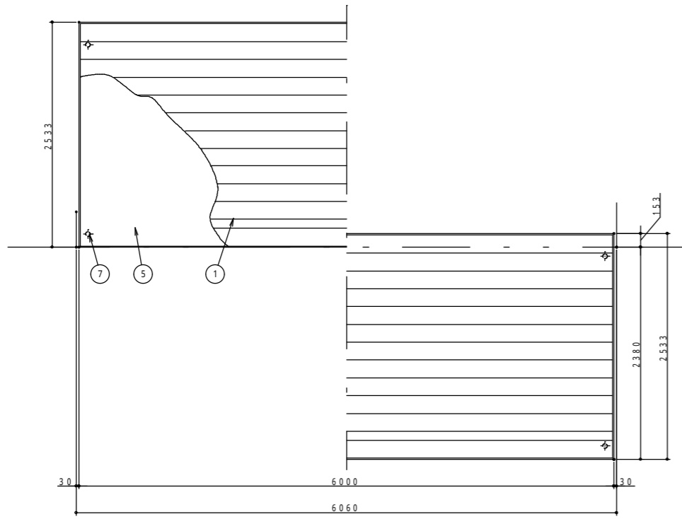
収納時平面図
