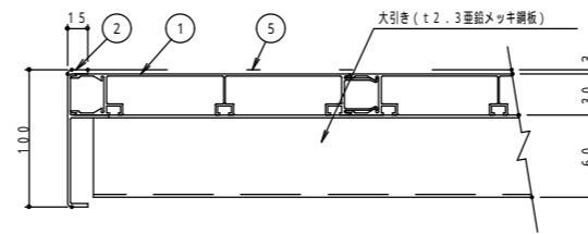
A部断面図 S = 1 / 3
