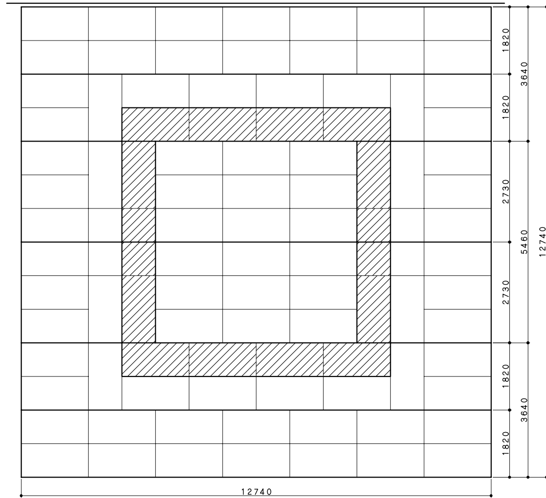
平面図 (98帖 略式サイズ)
