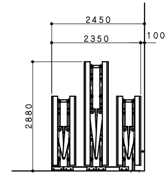
収納側面図 (98帖 略式サイズ)
