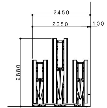
収納側面図 (98帖 略式サイズ)
