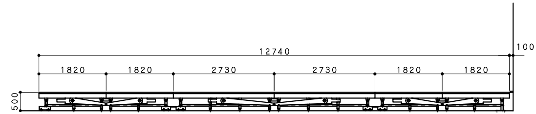
展開側面図 (98帖 略式サイズ)
