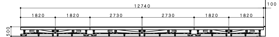
展開側面図 (98帖 略式サイズ)
